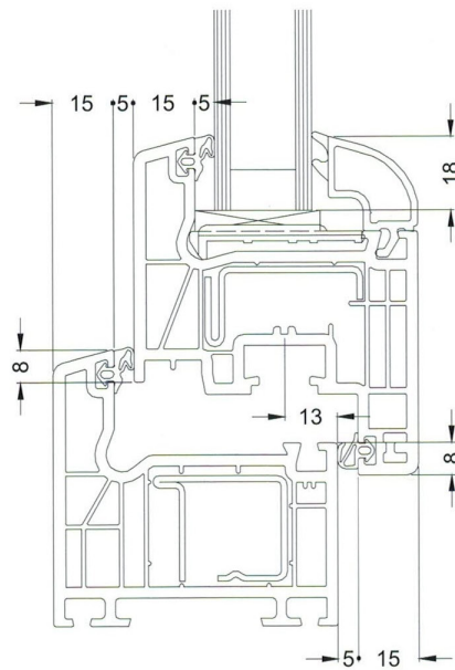
Sezione Schüco Corona CT 70 AS Classic
